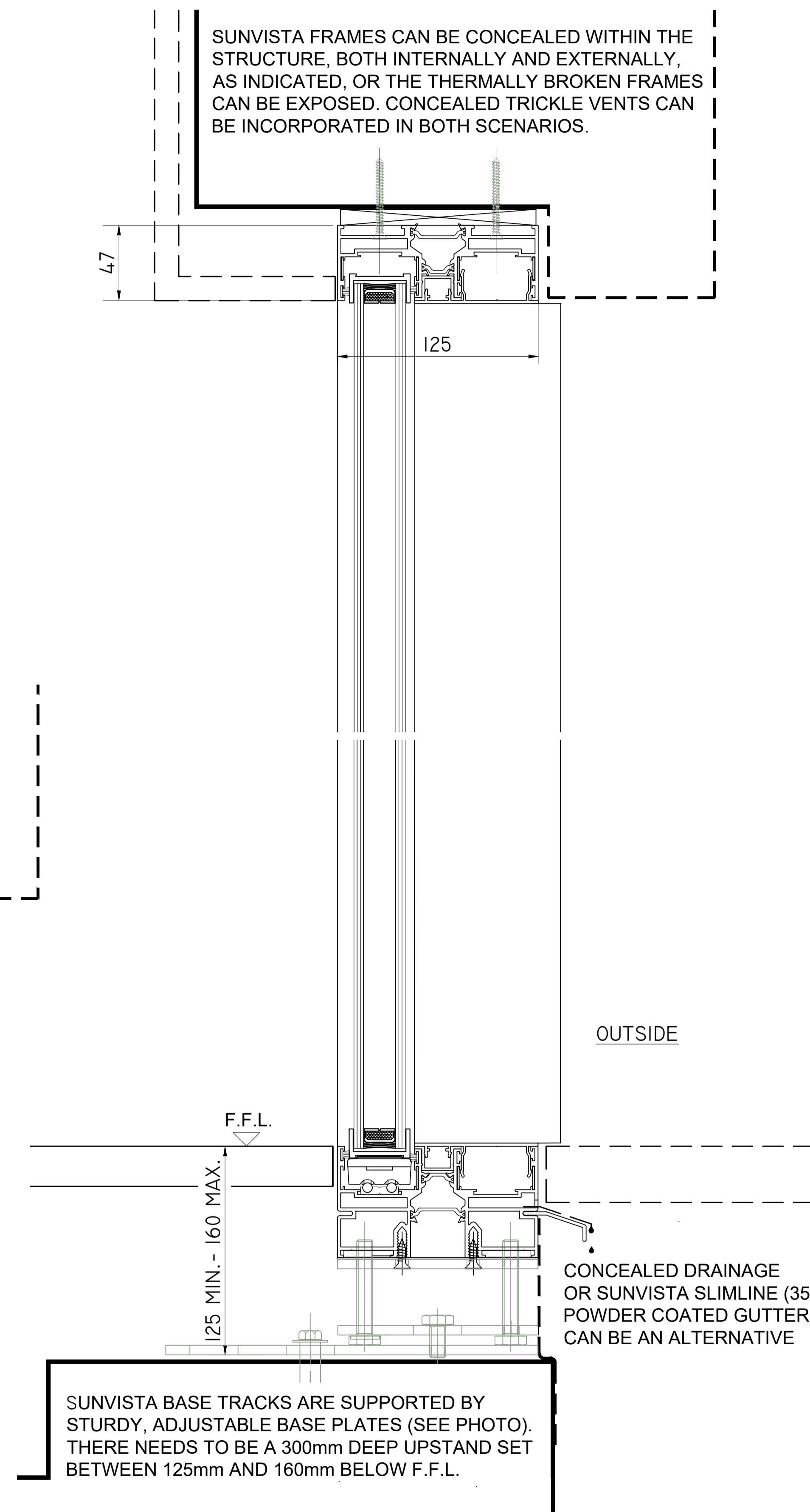
SECTION B.
